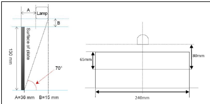
Anbau nach Zulassung Kategorie 1 (Kennzeichengröße: 240 x 130mm) Installation in compliance to category 1 (Licence plate size: 240 x 130mm)
