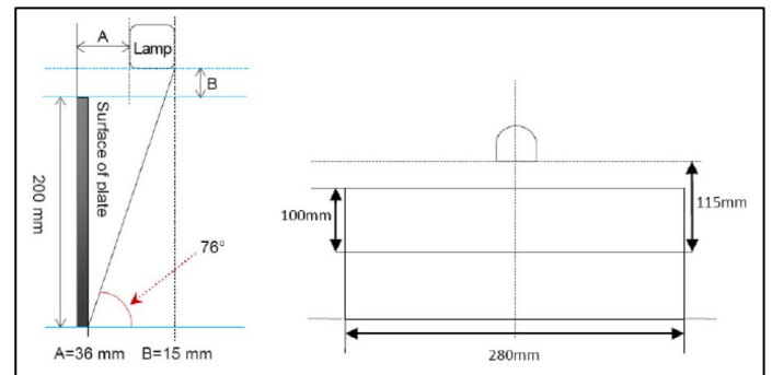
Anbau nach Zulassung Kategorie 2 (Kennzeichengröße: 280 x 200mm) Installation in compliance to category 2 (Licence plate size: 280 x 200mm)
