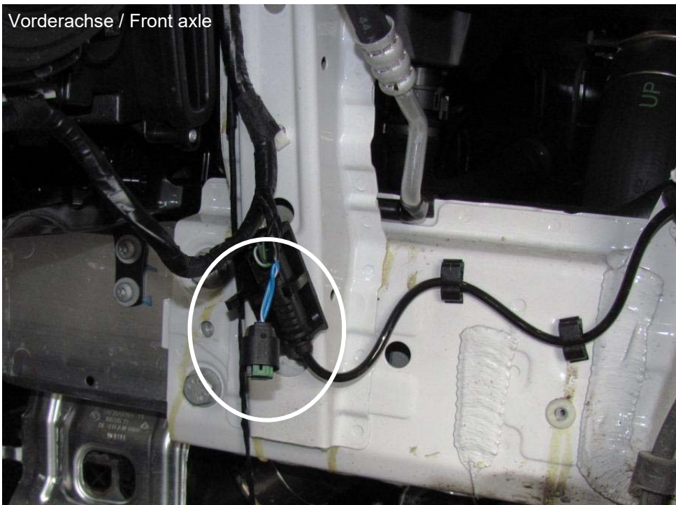
Steckersicherung
